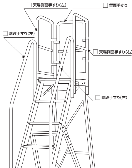
手すり取付け例
